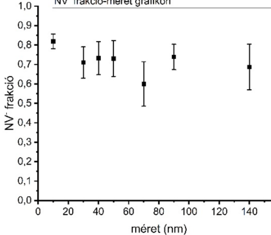
850°C-on 10 percig izzított COOH terminált minta: NV - frakció-méret grafikon
