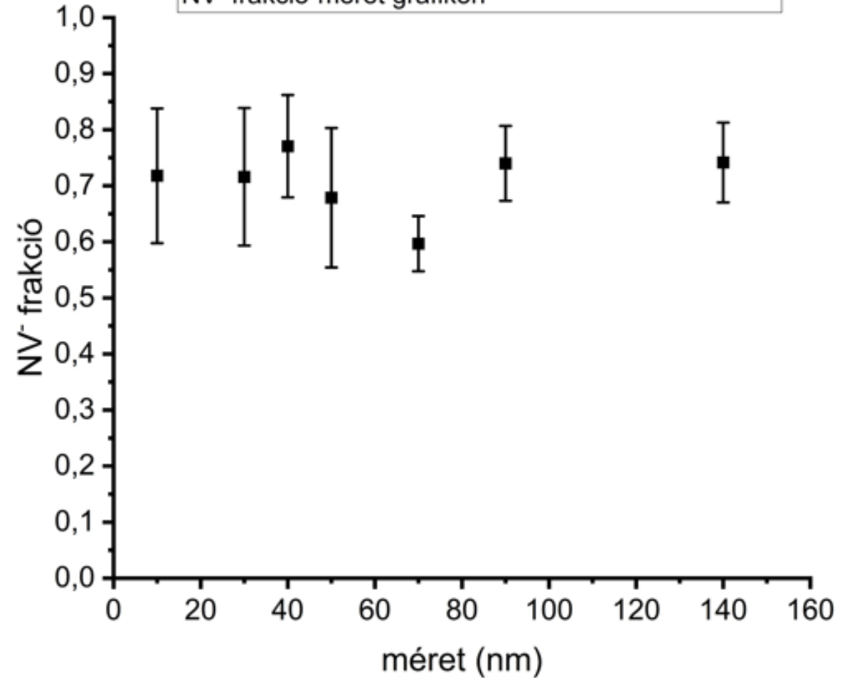
750°C-on 10 percig izzított COOH terminált minták NV - frakció-méret grafikon
